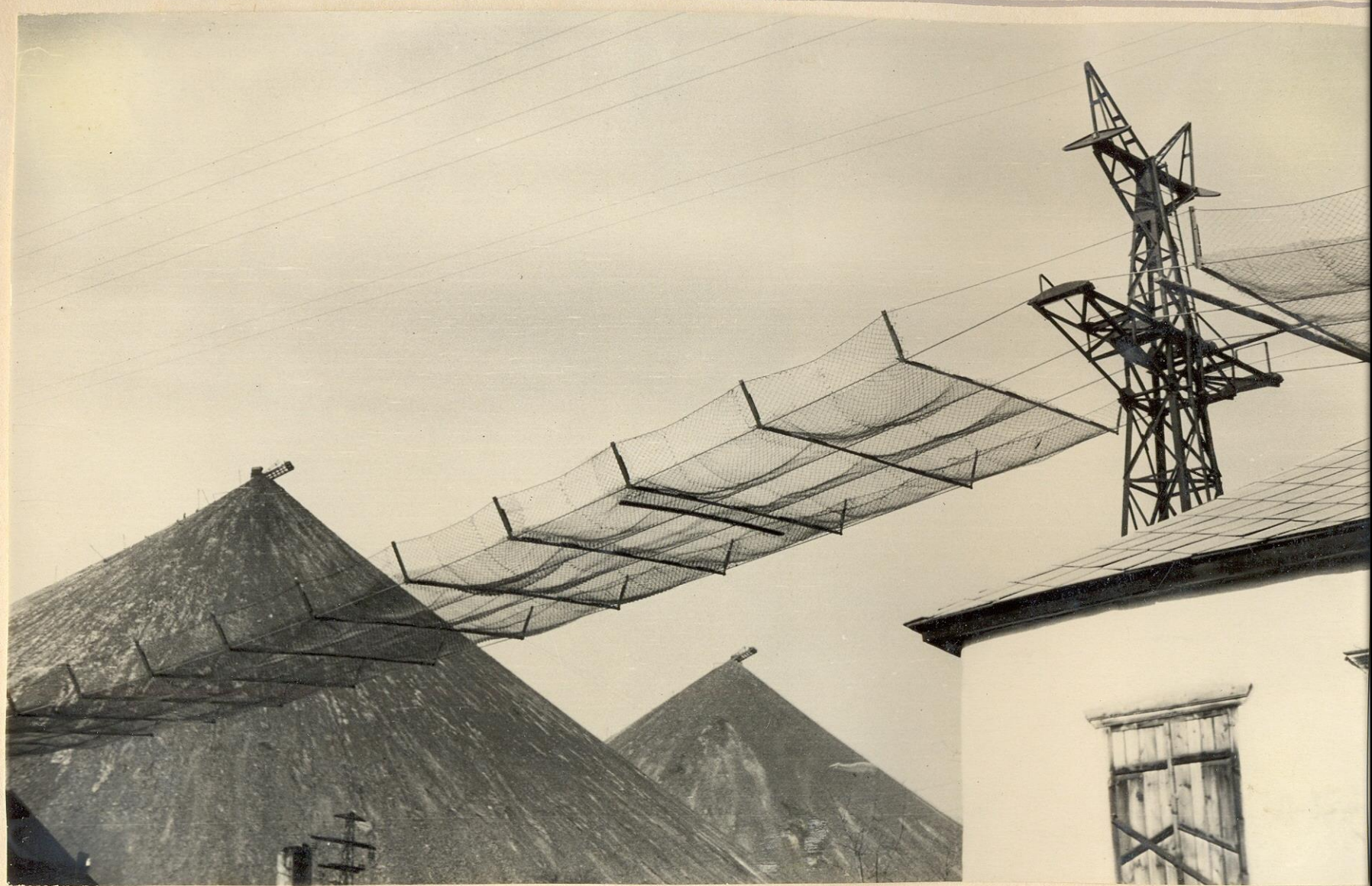
СТРОИТЕЛЬСТВО КАНАТНОЙ ДОРОГИ НА ШАХТЕ „КУЧЕГАРКА“
